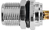
M8 母头面板式，焊接型，前锁安装
