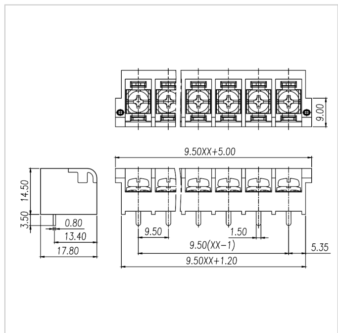
尺寸图
