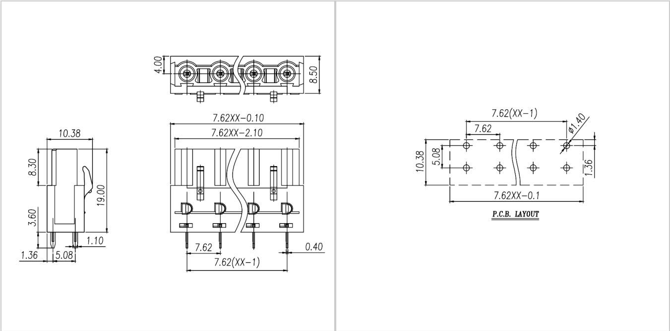
尺寸图
