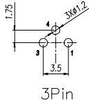
3Pin
