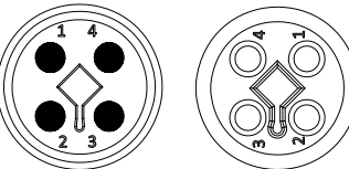
4PIN T-Coding
