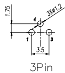
3Pin
