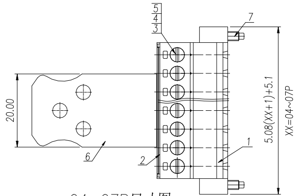
04~07P尺寸图
