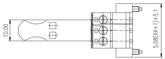
02~03P尺寸图
