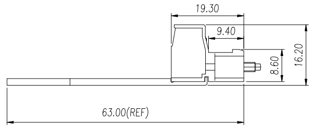
08~24P尺寸图
