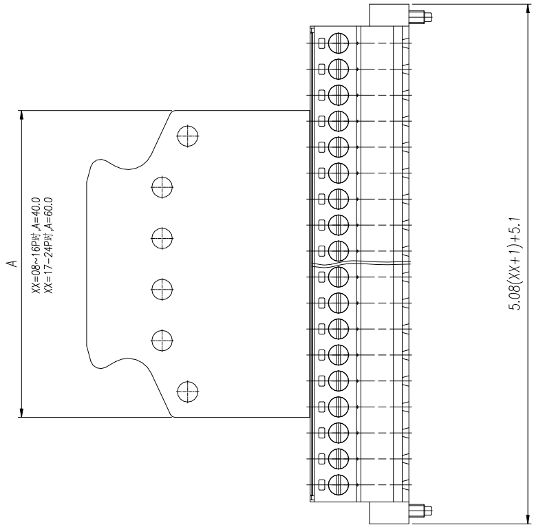
08~24P尺寸图
