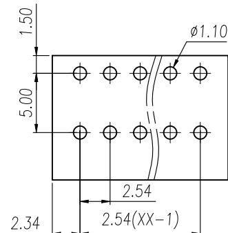
P.C.B. LAYOUT
